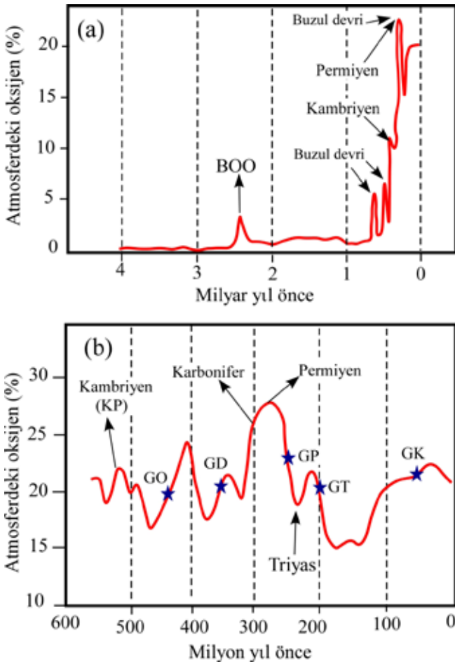
Şekil 5. Atmosferdeki oksijen miktarının (%) jeolojik tarih boyunca değişimini gösteren çizelgeler (Ward ve Kirschvink 2015'den yeniden çizilmiştir). Prekambriyen atmosferindeki oksijen miktarının ölçümlerinde büyük belirsizlikler bulunmaktadır. Şekil b'deki yıldız işareti Geç Ordovisiyen (GO), Geç Devoniyen (GD), Geç Permiyen (GP), Geç Triyas (GT) ve Geç Kretase'de (GK) meydana gelen toplu yokoluşları göstermektedir.
